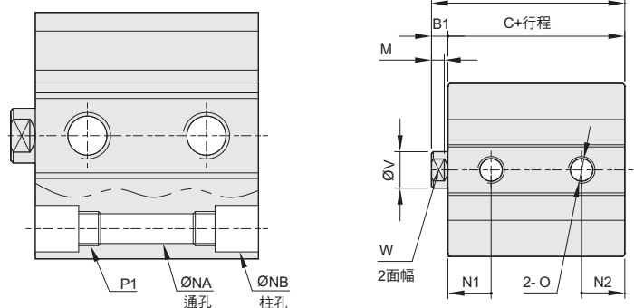
固定孔形式
